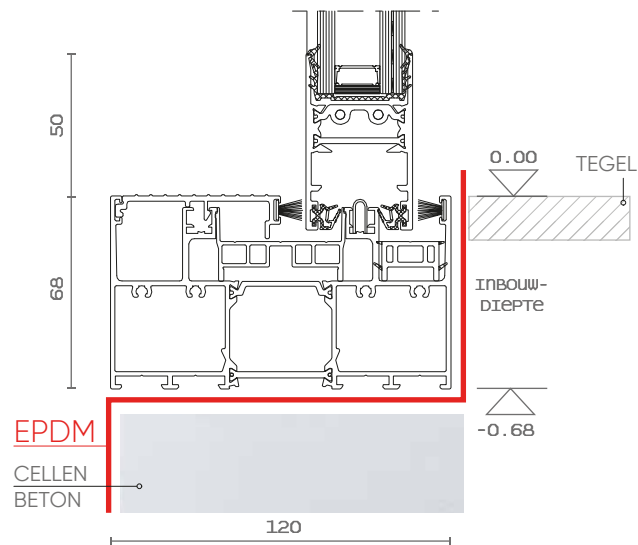
ONDER AANSLUITING
