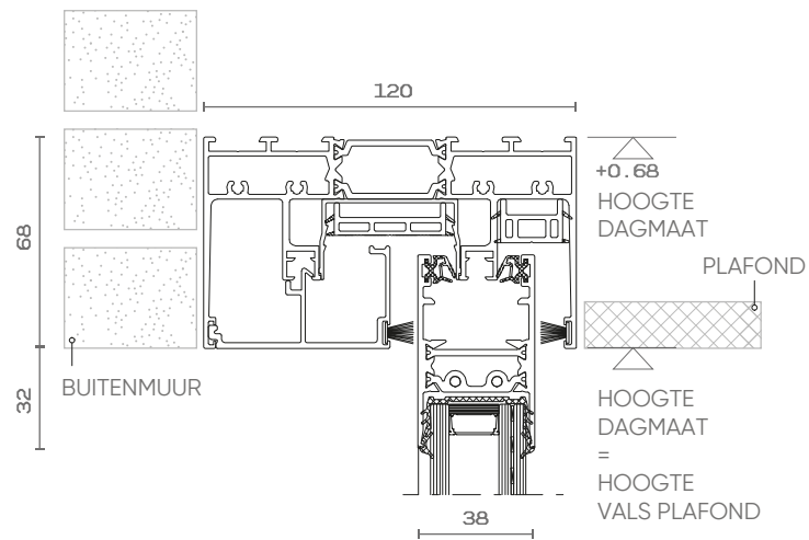
BOVEN AANSLUITING
