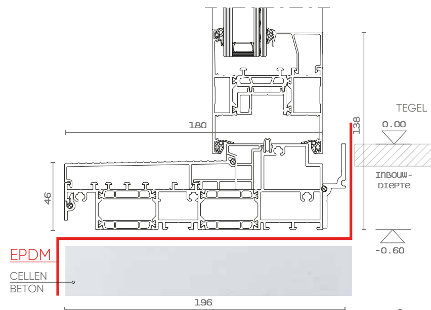
MONORAIL - ONDERAANSLUITING
